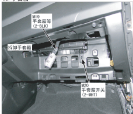
65. 手套箱
